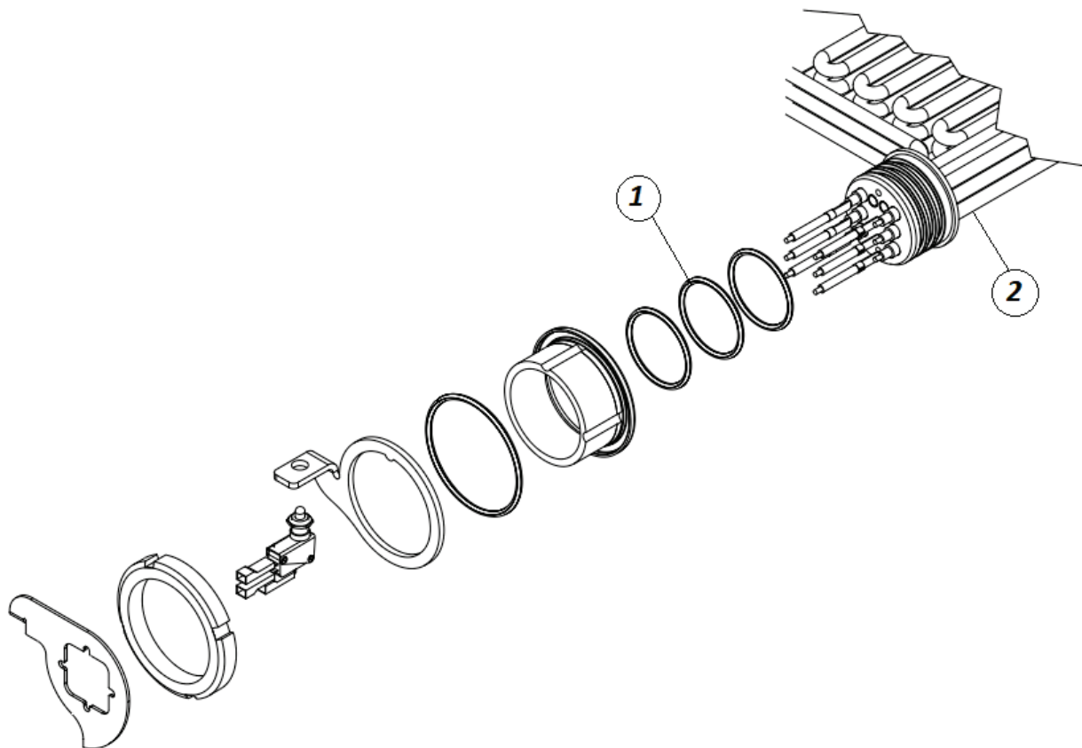
ABB. B (DREHWIDERSTAND)
